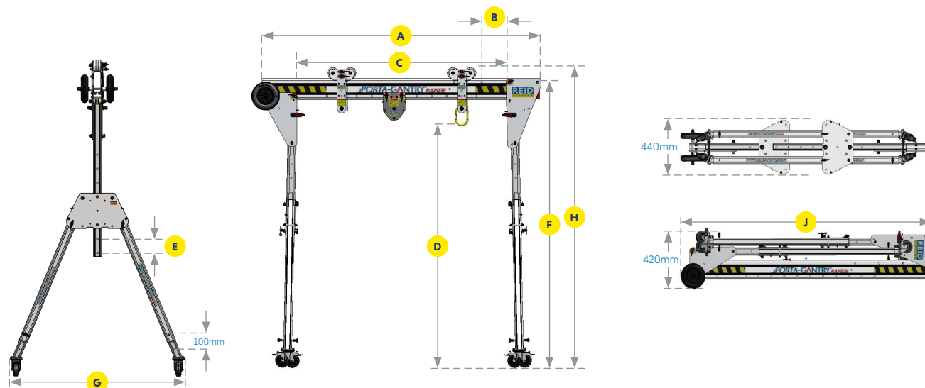
Afmetingen [mm]
