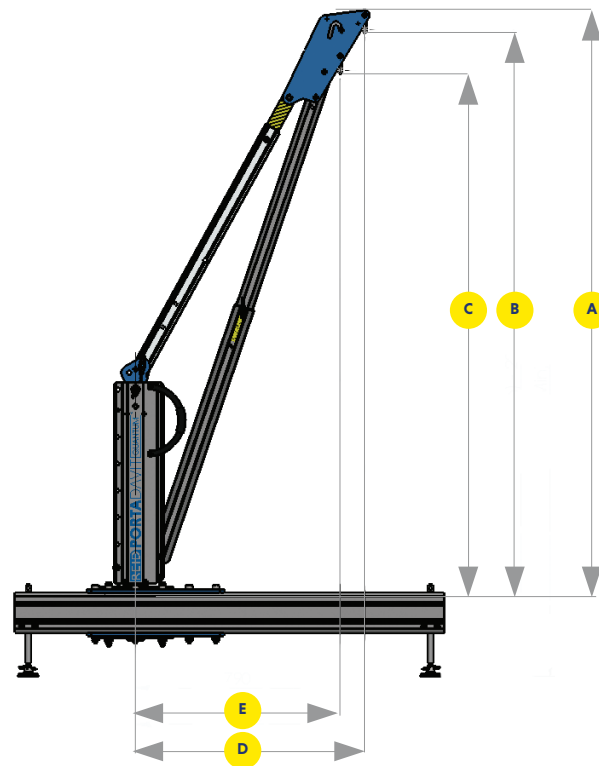
AFMETINGEN (MM)
