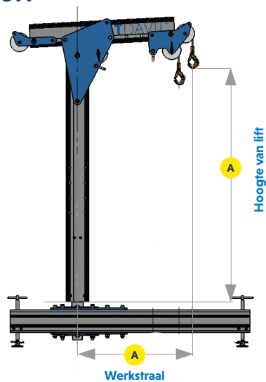
Positie A
