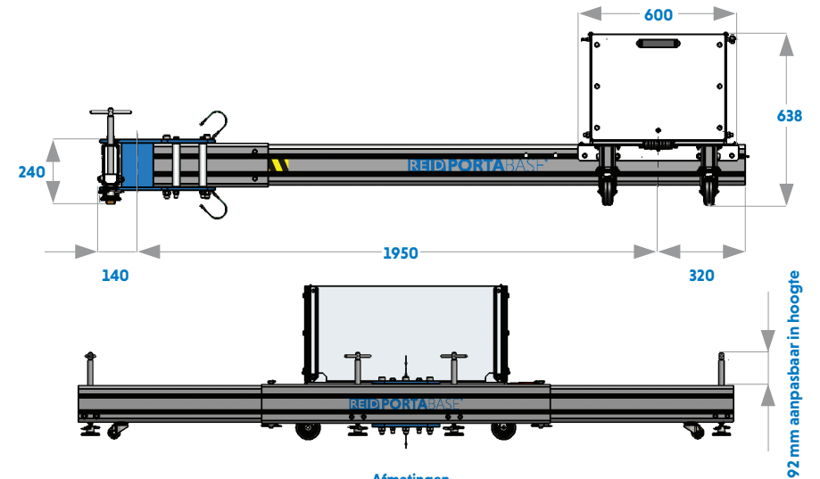
Afmetingen
