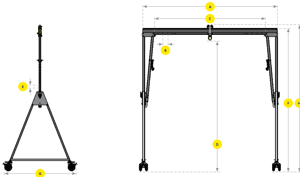
Standaardafmetingen balk
